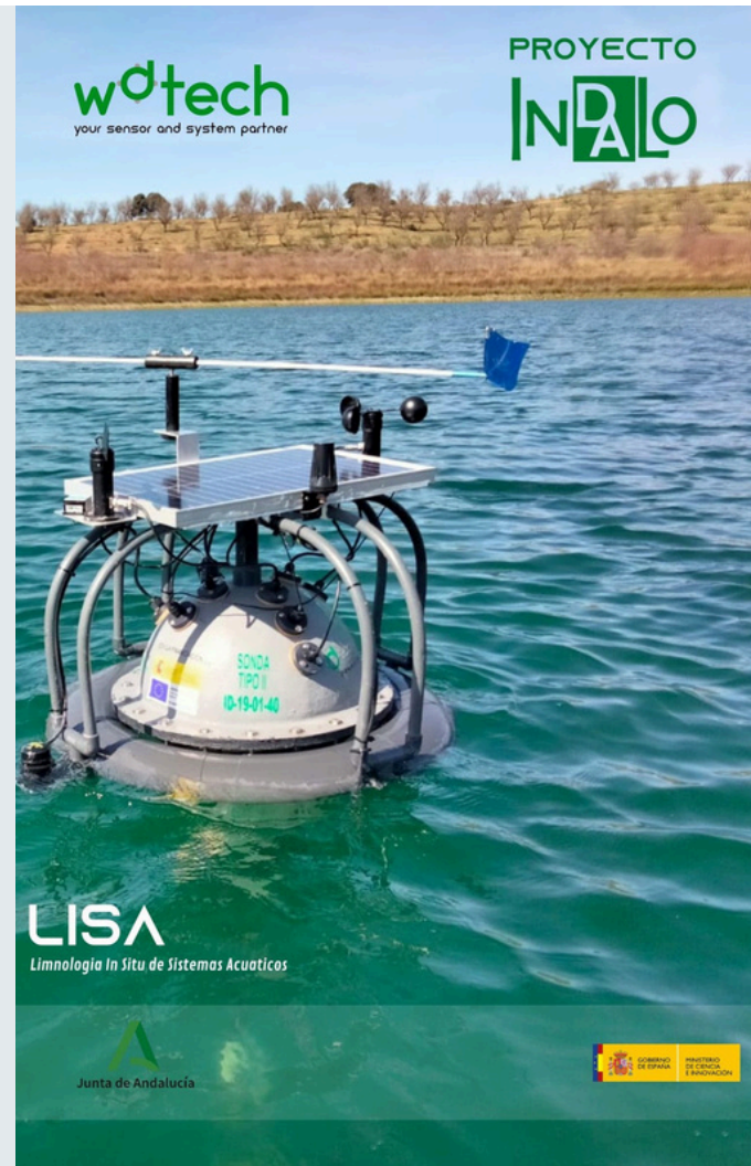
Sistema autónomo IOT de sondas con sensores multiparamétricos. LISA.
