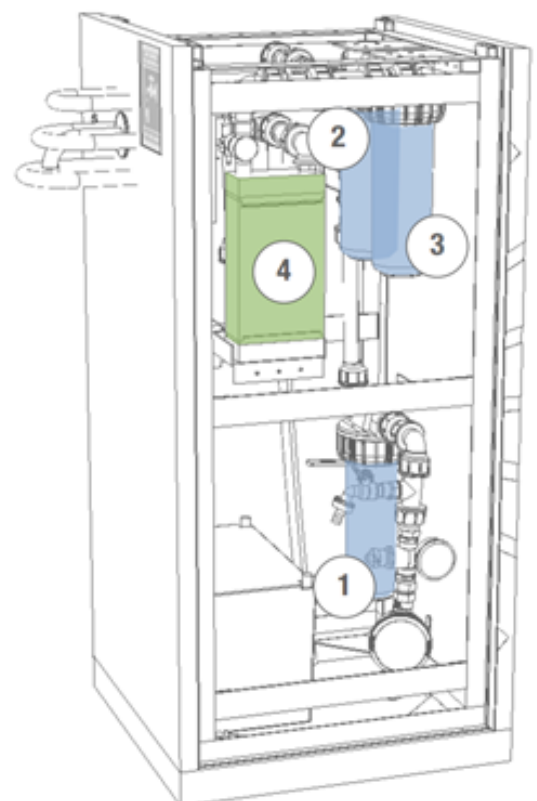
Figura 1. Esquema de la solución: 1, 2 y 3 (filtros de cartucho de 100 micras, 10 micras y carbón activo), 4 (germicida UVC)
