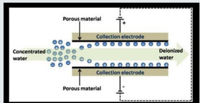
Figura 1. Esquema del proceso de Desionización Capacitiva (CDI)
