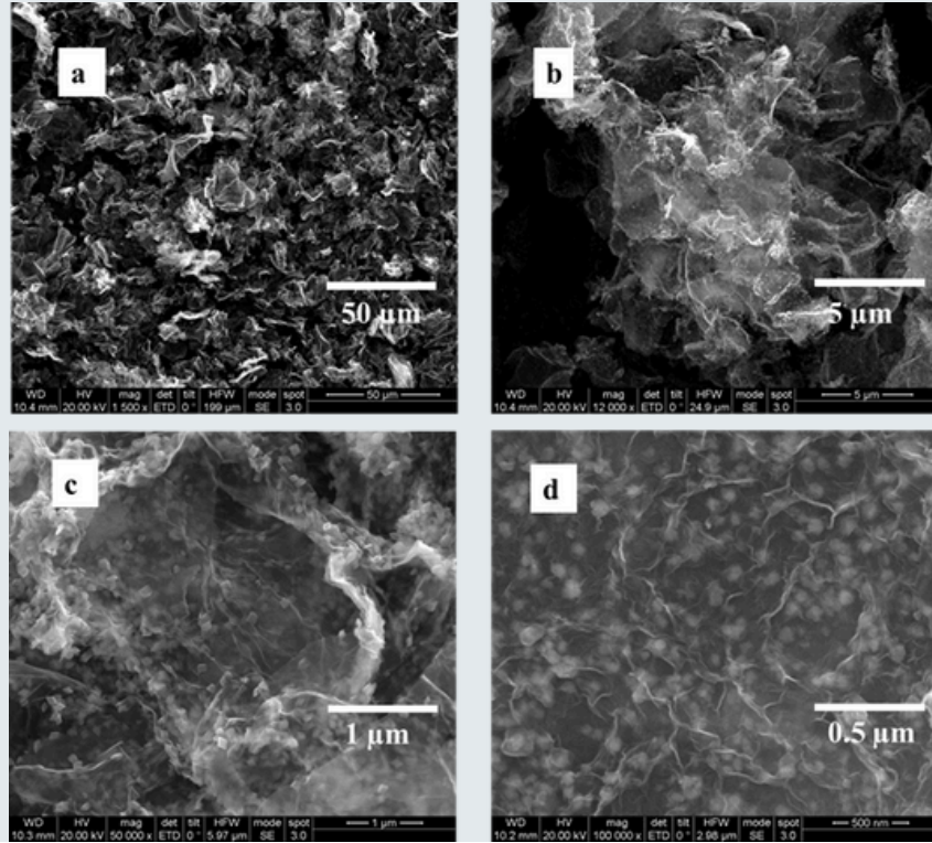
Figura 2- SEM del compuesto de grafeno a varias magnificaciones
